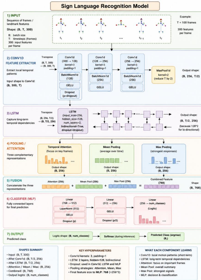
Figure 8: معمارية النموذج المقترح
