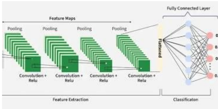
Figure4: آلية عمل الشبكات العصبية الالتفافية
